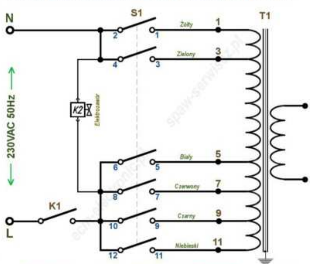
Schemat zasilania transformatora spawarki typu XTE181C
